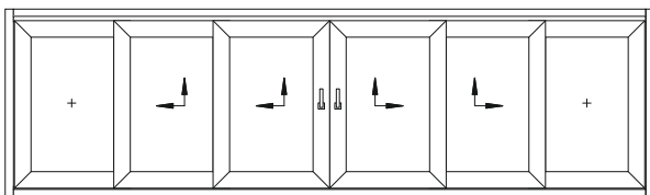
Beschlagschema L
