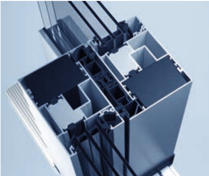
heroal S 77 HI, Mittelstoß mit vier Dichtebenen und Windstop
