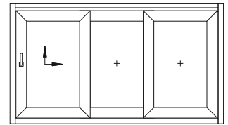
Beschlagschema A
