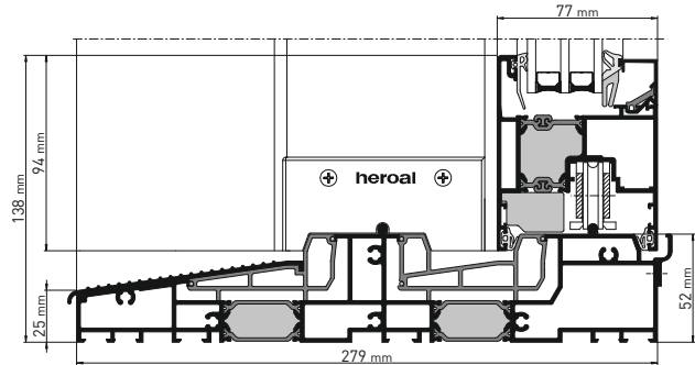
heroal S 77 HI, 3-spurig, Schnittdarstellung
