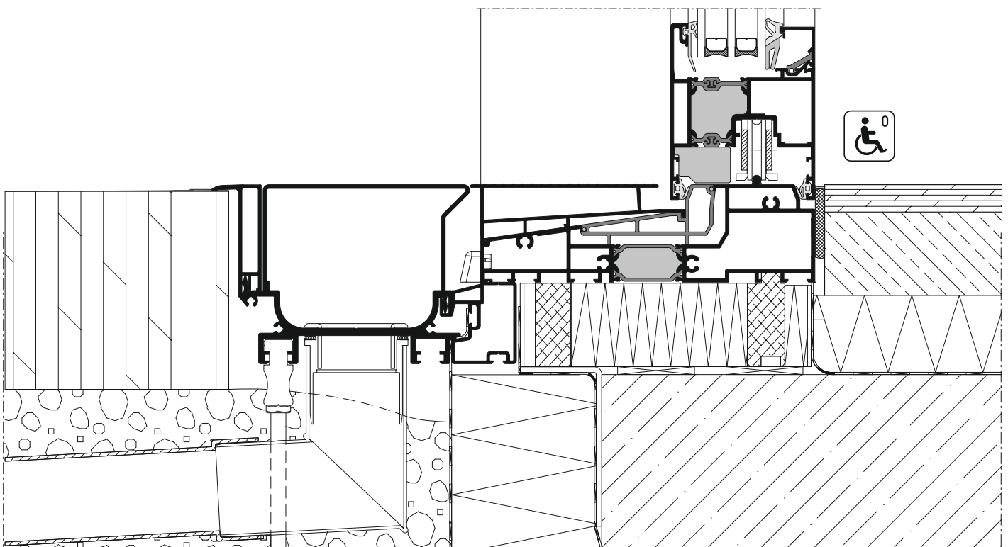
heroal S 77, Null-Barriere nach DIN 18040, Schnittdarstellung
